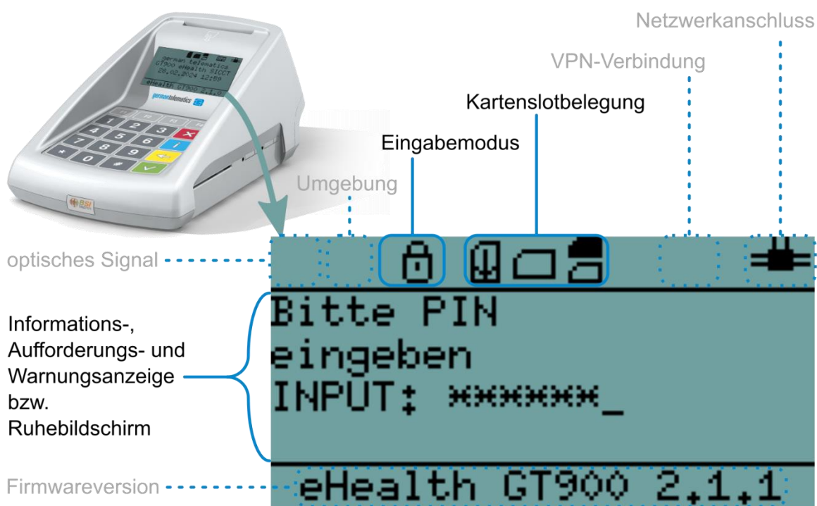
Abbildung 16: Mögliche Displayanzeige des Kartenterminals bei der Eingabe einer Karten-PIN. In diesem Beispiel wird die Karten-PIN an die Karte im eGK-Slot gesendet (zusätzlich sind eine Karte im eHBA/SMC-B-Slot und eine gSMC-KT eingelegt).
