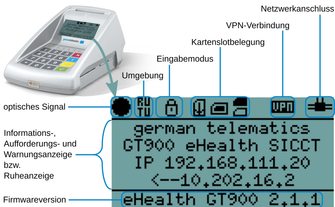
Abbildung 13: Displayaufbau des eHealth GT900 Kartenterminal
