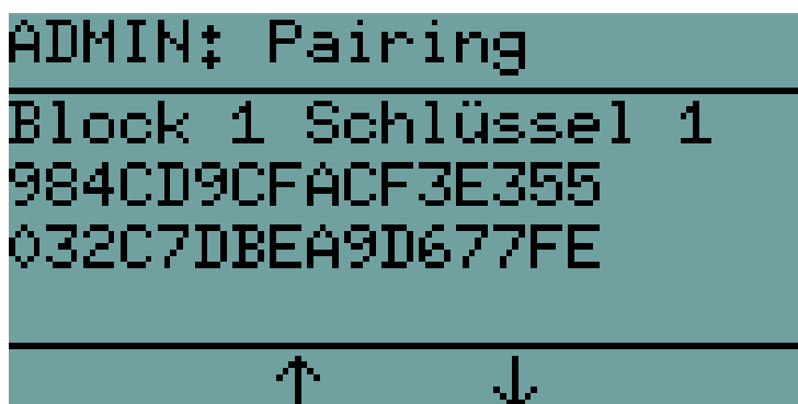
Abbildung 32: Menü zum Anzeigen vorhandener Fingerprints
