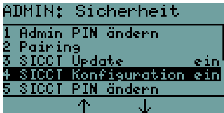
Abbildung 39: Anzeige des Submenüs "Sicherheit"
