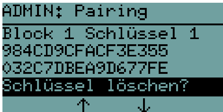
Abbildung 35: Menü zum Löschen von Pairing-Schlüsseln
