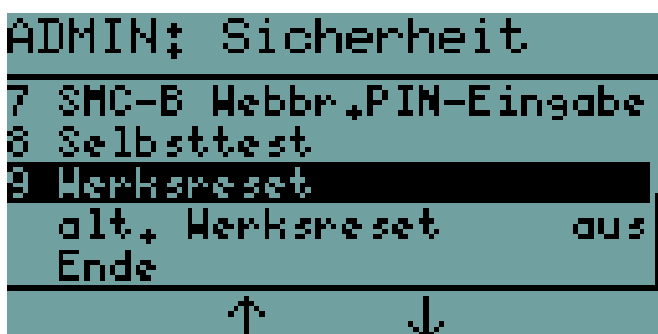
Abbildung 69: Anzeige des Submenüs "Sicherheit"
